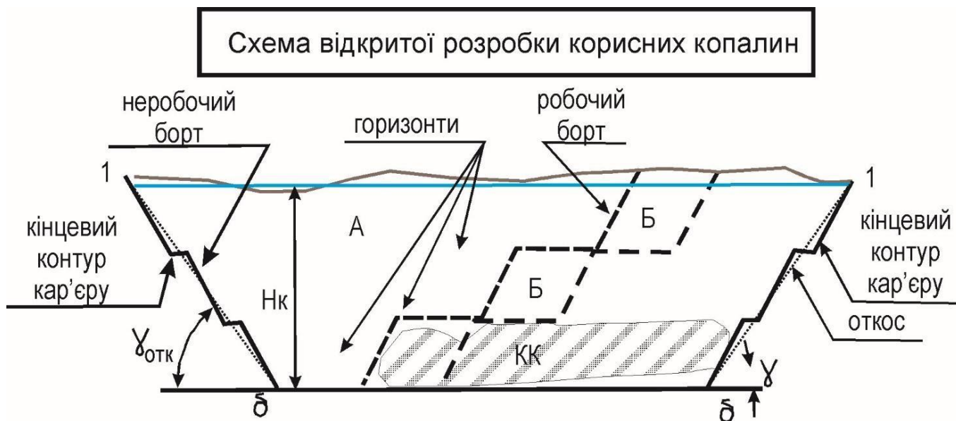
Рис. 1. Схема відкритої розробки КК
